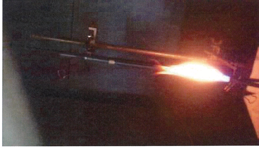
自己消火性の実証試験の例（UL垂直燃焼試験）
